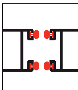
Doble junta Marcos de 42 mm
