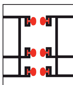
Triple junta Marcos de 60 mm
