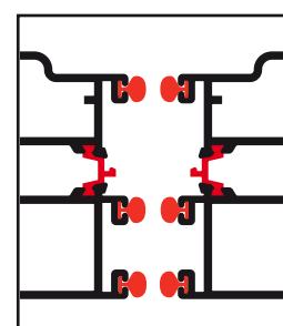
RPT (rotura de puente térmico) Marcos de 80 mm
